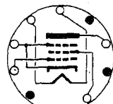
EL84
