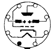
EM34
