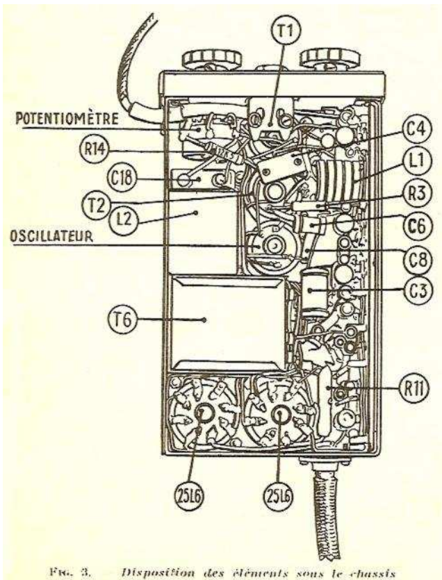
FIG. 3. Disposition des éléments sous le châssis
