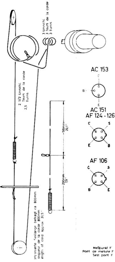
Seilschema Schema pour le montage de la corde d'accord Drive cord diagram
