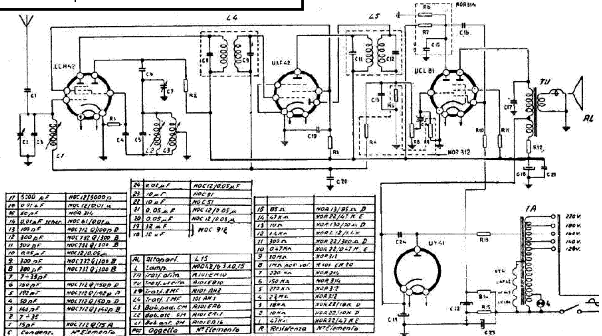
TELEFUNKEN (COMPAGNIA RADIORICEVITORI) - Mod. Mignonneite Baby. Onde medie con sintonia a permeabilità variabile. Media frequenza 468 kc/s. Tensione al primo elettrolitico 160 V e 140 V al secondo. Potenza di uscita 2,5 watt. Consumo 30 watt.
