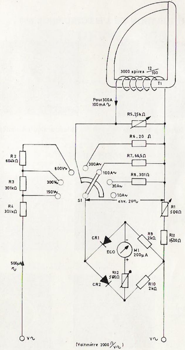
ELECTROPINÇE 400 SCHEMA DE PRINCIPE
