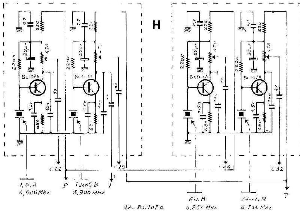
Fig. IV-3. — Les oscillateurs de fréquence zéro et d'identification.
