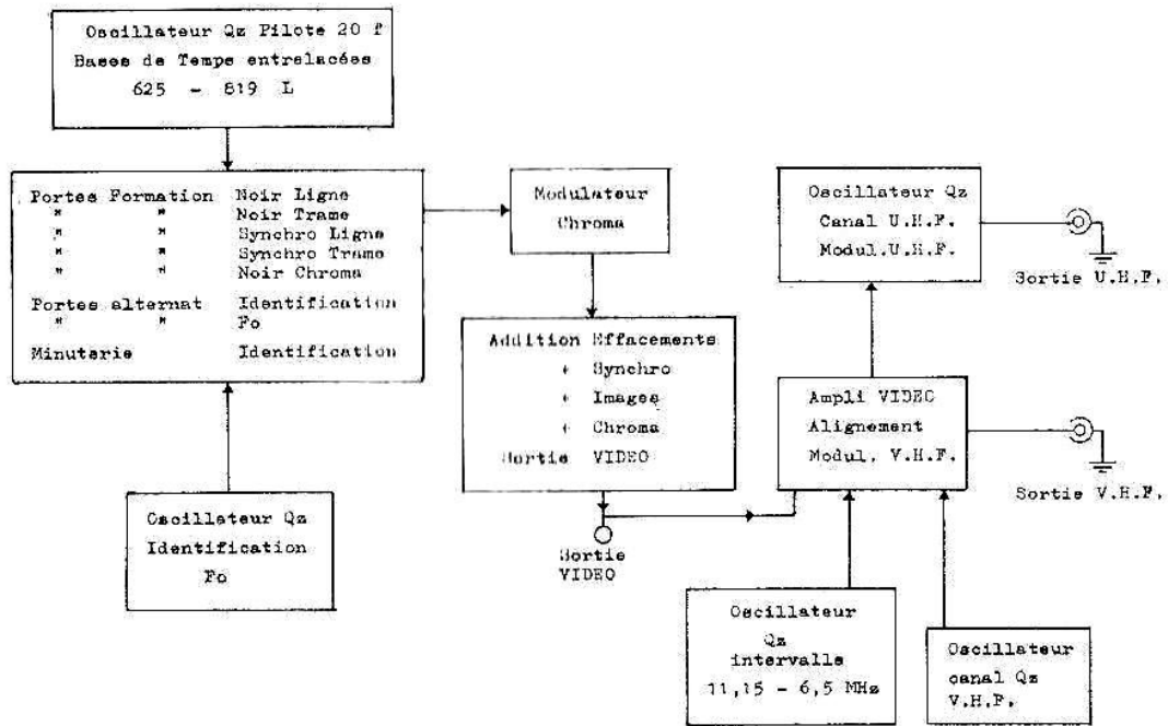
Fig. IV-2. — Schéma-bloc de la mire.
