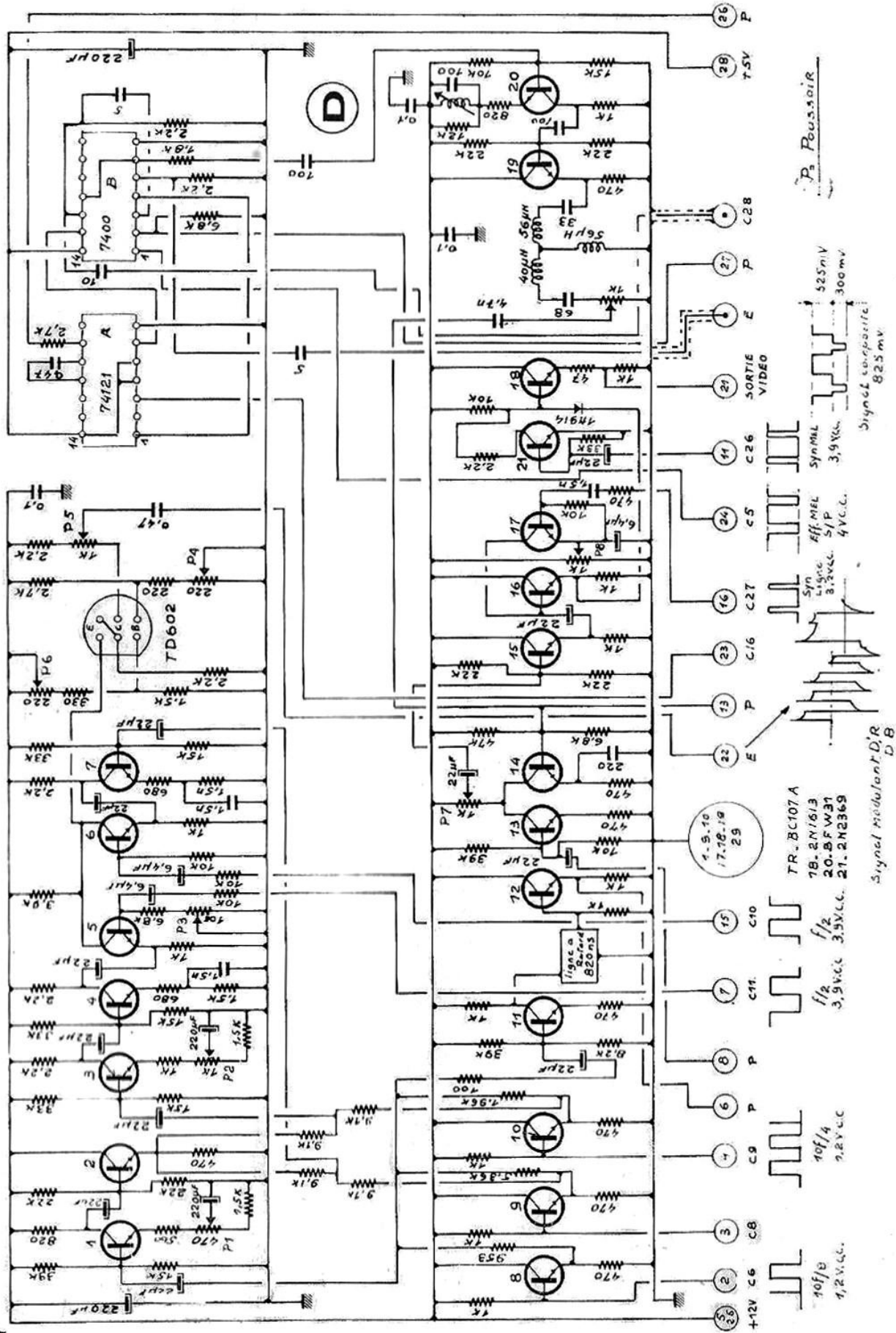
Fig. IV-7. — Les étages d'élaboration des signaux de service.
