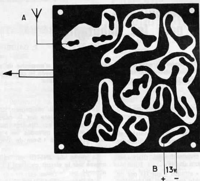
Convertisseur. Circuit imprimé vu côté cuivre
