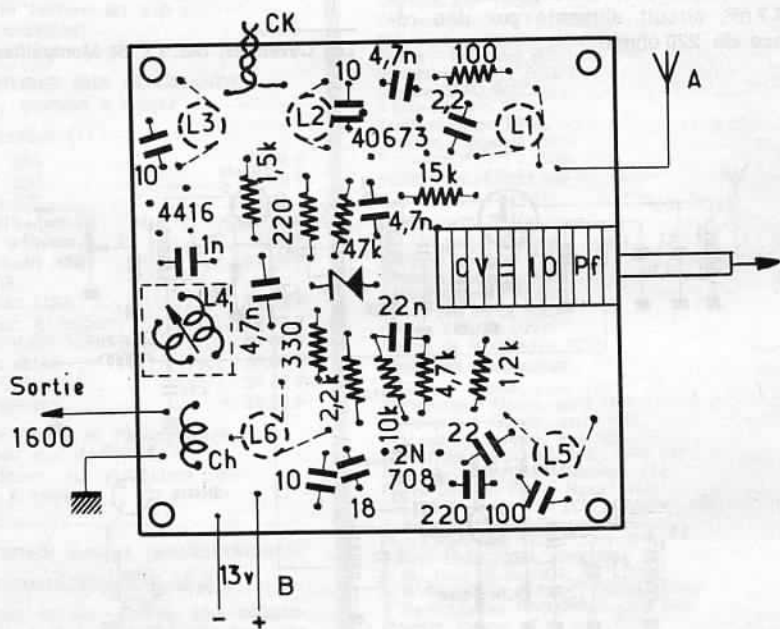
Convertisseur. Circuit vu côté composants
