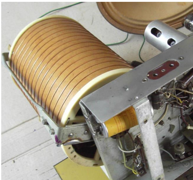
Antenne cadre
