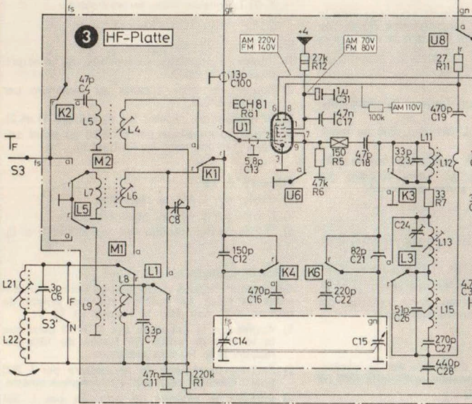
Ferrit-Antenne Ferrite antenna Cadre ferrite
