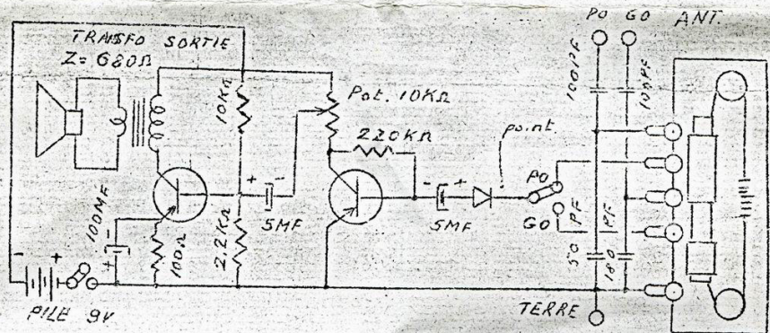
2 TRANSISTORS avec HAUT PARLEUR
