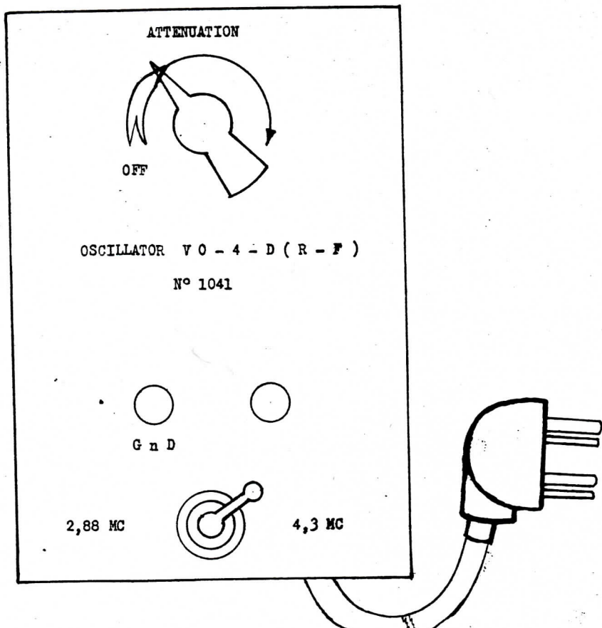
Fig. 30 a. Vue du panneau avant du V 0 - 4 - D Zicht op voorpaneel V 0 - 4 - D
