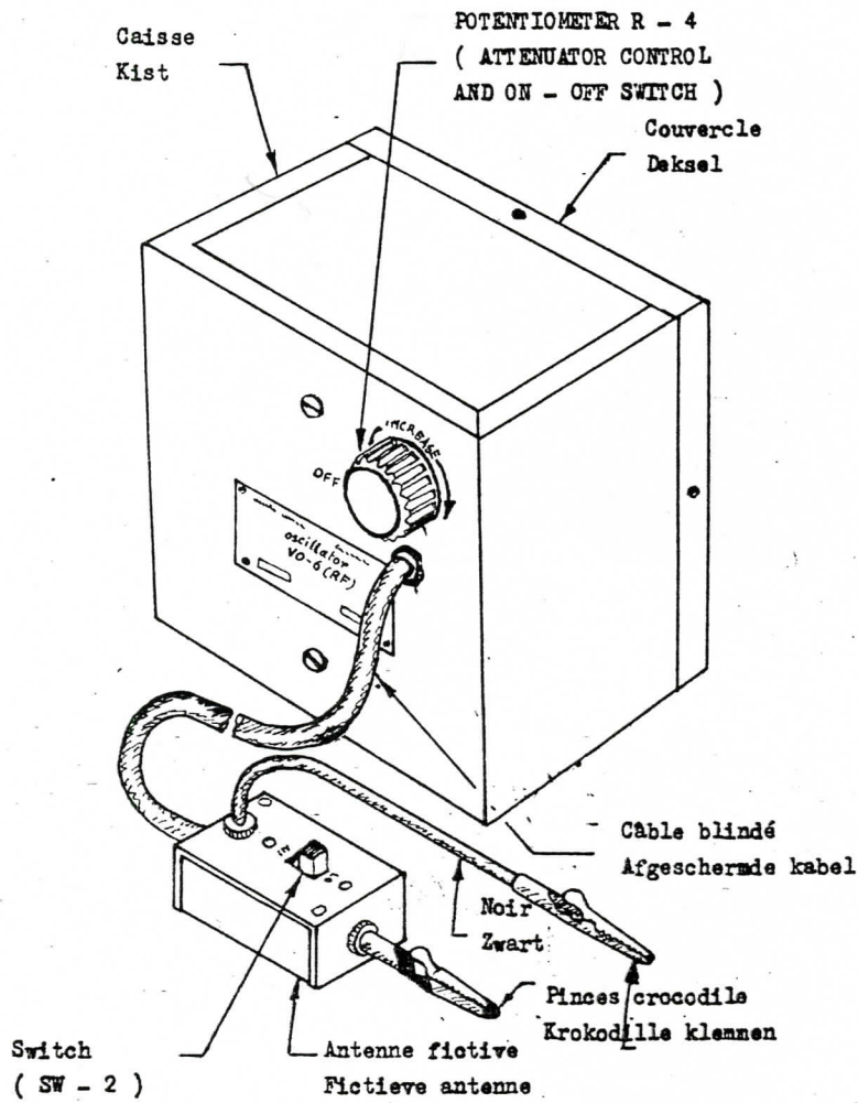
Fig. 31. Vue du panneau avant du V O - 6 Zicht op het voorpaneel van de
