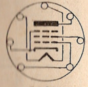
6AQ5
