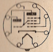
ECH42
