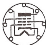
6BA6
