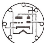
6AV6
