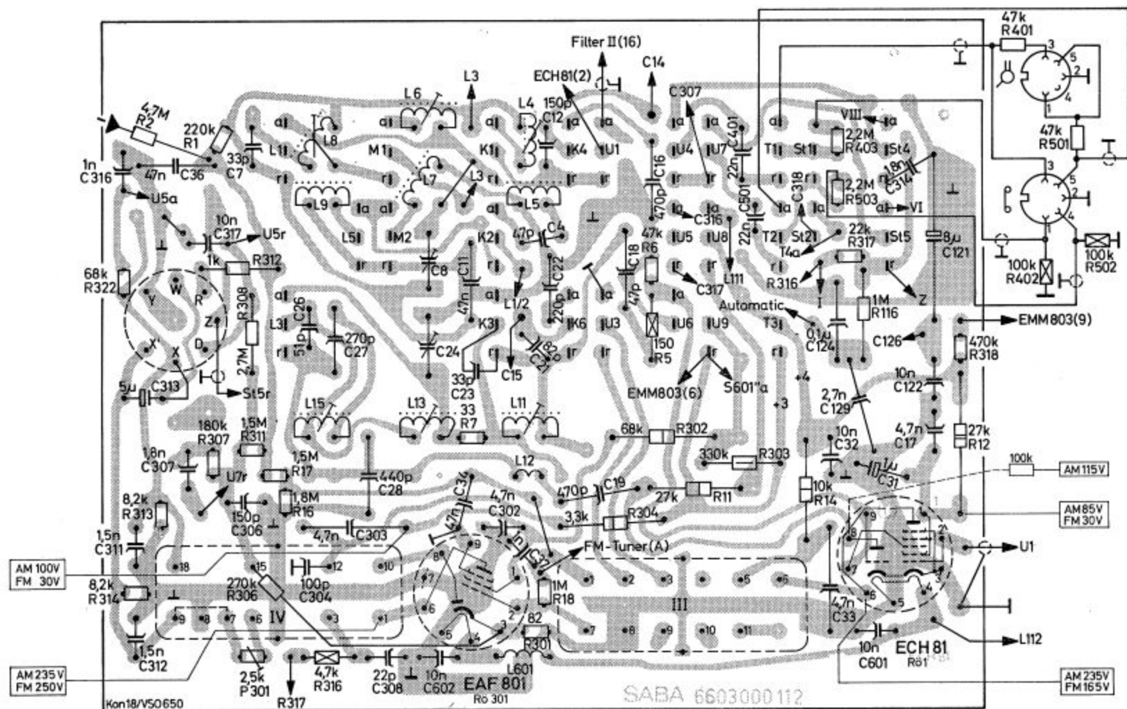
HF-Platte
