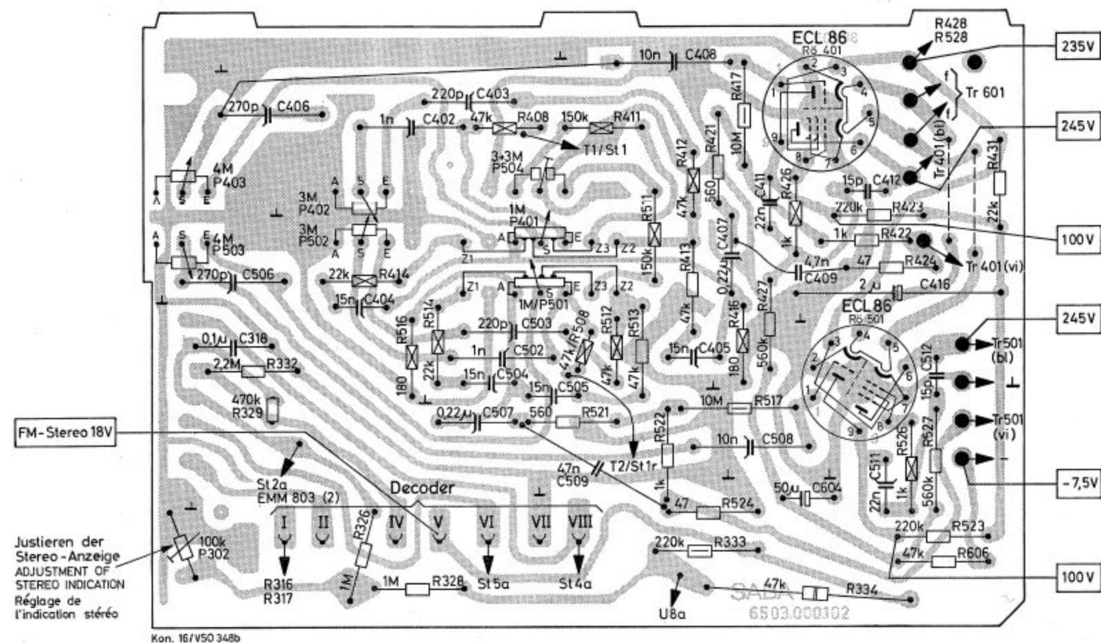
NF-Platte
