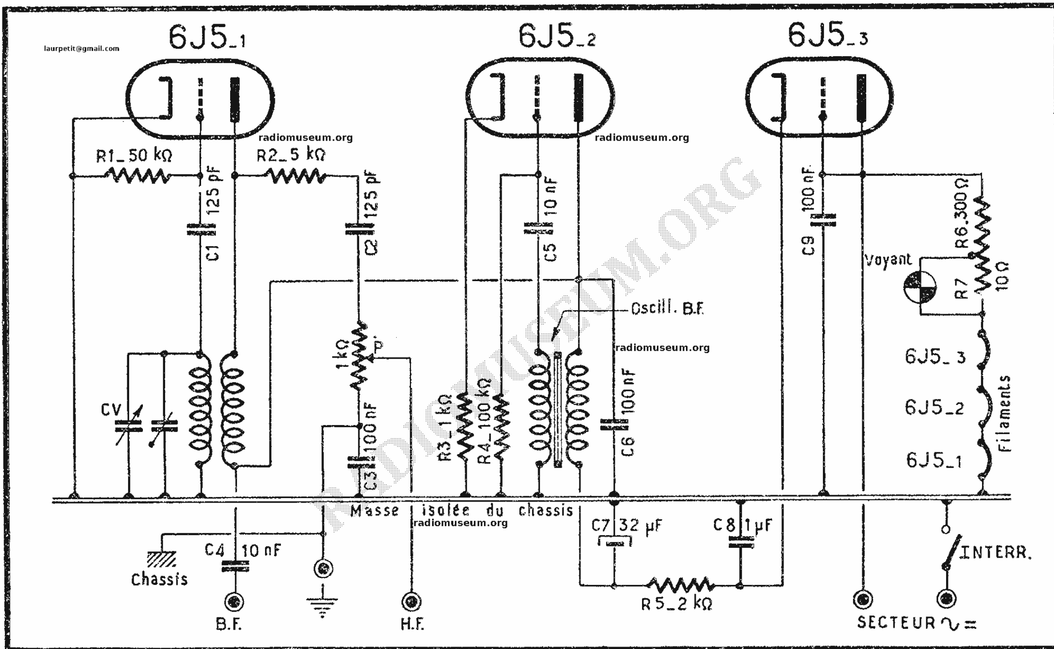
Schéma général du générateur A-45.
